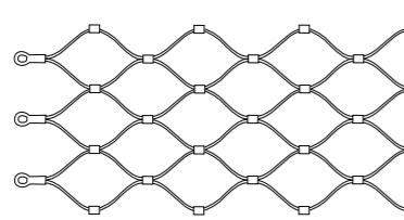
X-TEND, Randausbildung mit Ösen X-TEND, Edging with eyelets
