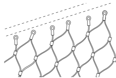
X-TEND, Schrägnetz - Montage mit Ösen X-TEND, diagonal mesh - Installation with eyelets
